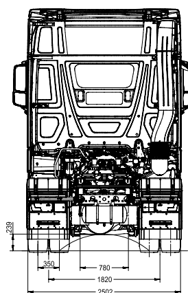
后视图
