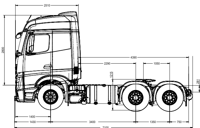
侧视图
